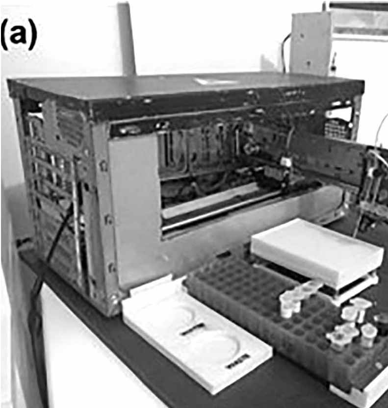
Versões do analisador: na foto (a), versão inicial, utilizando partes recicladas de computadores e impressoras convencionais; em (b), a versão atual, utilizando impressoras 3D
