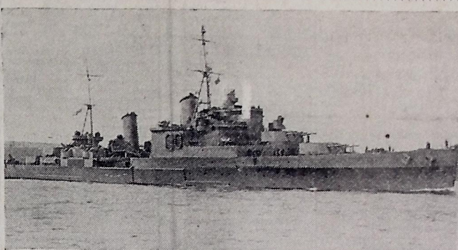
O "H. M. S. Newcastle", cruzador britânico da Classe do "Southampton", terminado em 5 de março de 1937. Deslocando 9.100 toneladas, o "Newcastle" é armado com 12 peças de 6 polegadas, 8 de 4, além de 6 tubos lança-torpedos. Conduz a bordo um avião, lançado por meio de catapulta, e com uma equipagem de 700 homens. (Foto do British News Service para a UNIAO)
