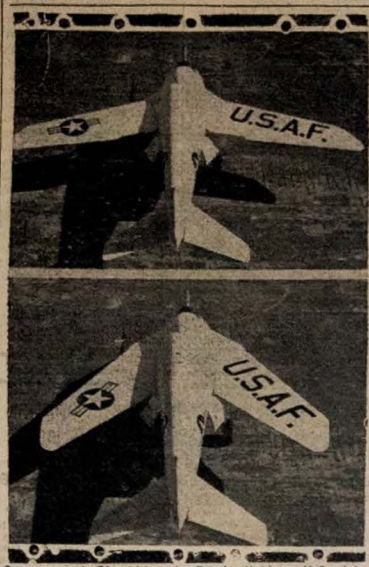
O novo caça da Força Aérea dos Estados Unidos, o X-5, a jato, equipado com asas móveis, que podem ser ajustadas pelo piloto em pleno voo. Sua velocidade a grandes altitudes é a maior jamais registrada por qualquer avião de mesmo tipo. Na foto, vê-se o X-5 com as asas na posição avançada, para decolagem, elevação ou aterrissagem e com elas recuadas, que favorece o voo mais rápido. (foto USIS)
