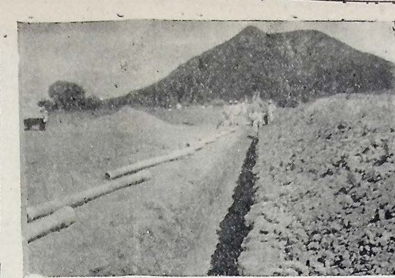
ADUTORA DE CATOLÊ DO ROCHA — O Governo do Estado, através do Departamento de saneamento, órgão da Secretaria de Viação, iniciou os trabalhos de construção da adutora que ligará o poço do Cajueiro (em Petrópolis) — cidade de Catolê do Rocha. Trata-se de um serviço cuja conclusão trará a solução ao problema do abastecimento d'água daquela cidade sertaneja. Na gravura, um flagrante dos trabalhos de construção da adutora.
